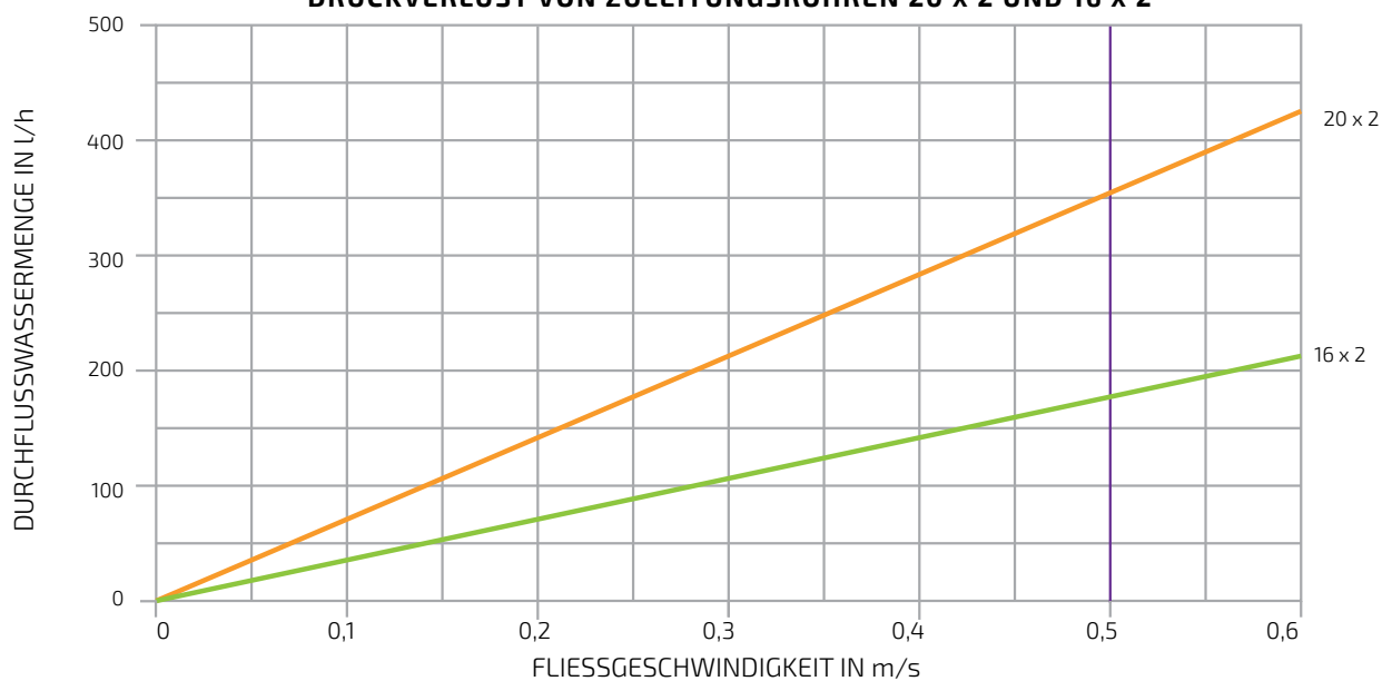
DRUCKVERLUST VON ZULEITUNGSROHREN 20 x 2 UND 16 x 2
