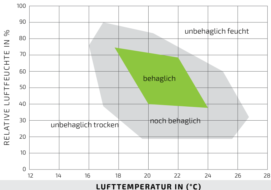
BEHAGLICHKEIT IN ABHÄNGIGKEIT VON LUFTFEUCHTE und -TEMPERATUR
