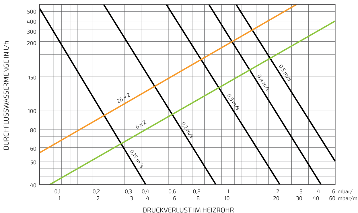
DRUCKABFALL DER ANBINDELEITUNGEN - ROHRE: 20 x 2 UND 16 x 2
